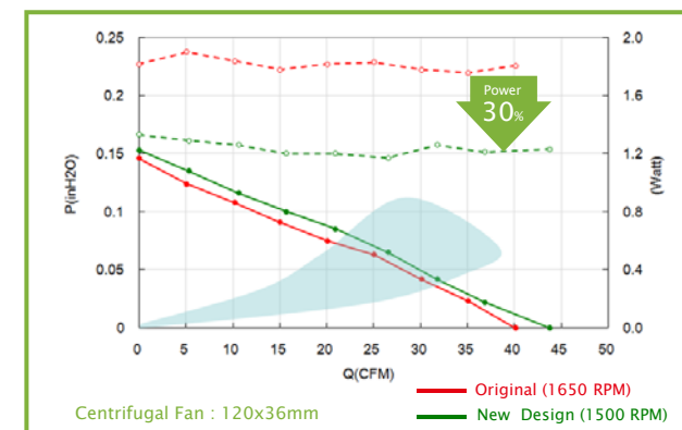
Centrifugal Fan : 120x36mm
